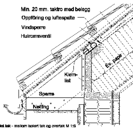
Montering i luftet tak - mellom isolert tak og ventiltak M 1:5
